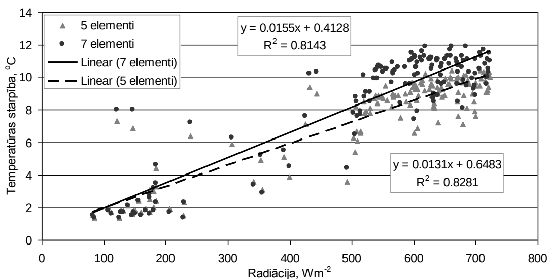
5.3. att. Temperatūras pieaugums gaisa sildīšanas saules kolektora izejā diviem dažādiem absorbentiem (5 un 7 elementi rindā) atkarībā no saules radiācijas
