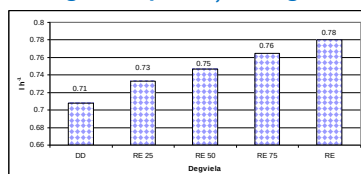
Degvielas patēriņš brīvgaitā
