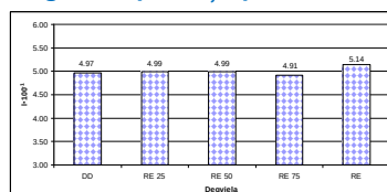
Degvielas patēriņš pie 90 km h -1
